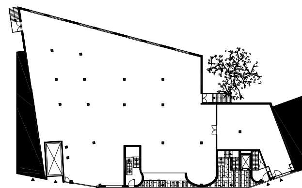
begane grond
